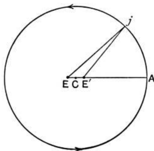
FIG. 35.—The equant.
