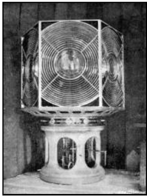
DIOPTRIC LANTERN.
