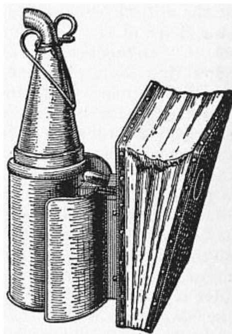
FIG. 26.—Bee-Smoker.
