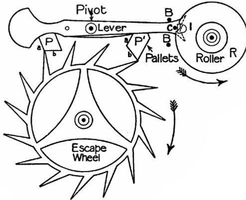
FIG. 205.—"Lever" watch escapement.
