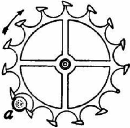
FIG. 204.—"Cylinder" watch escapement.
