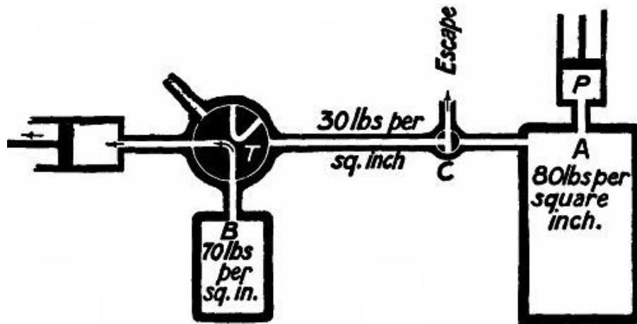
FIG. 89.—Brake "on."
