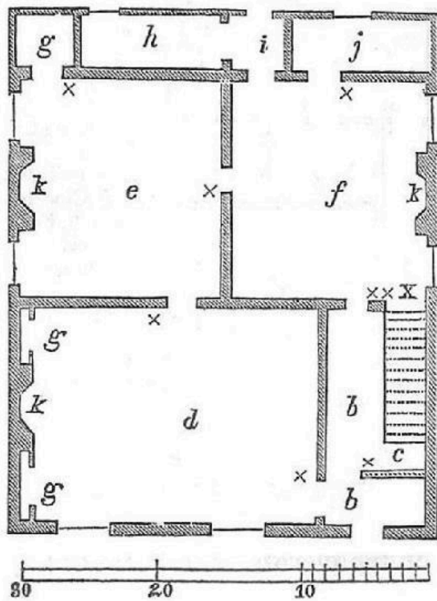
Fig. 27. Ground-plan.
