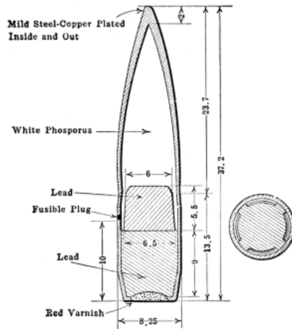
FIG. 111.—German 8" Incendiary Bullet.
