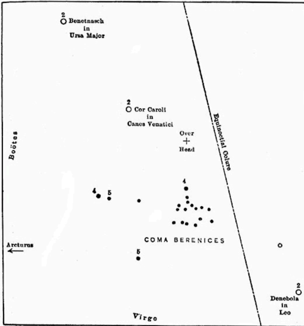
COMA BERENICES
