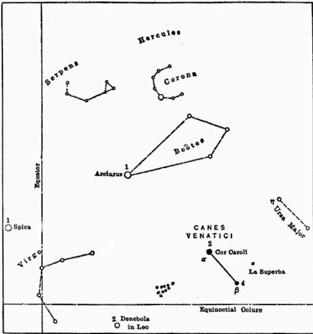
CANES VENATICI
