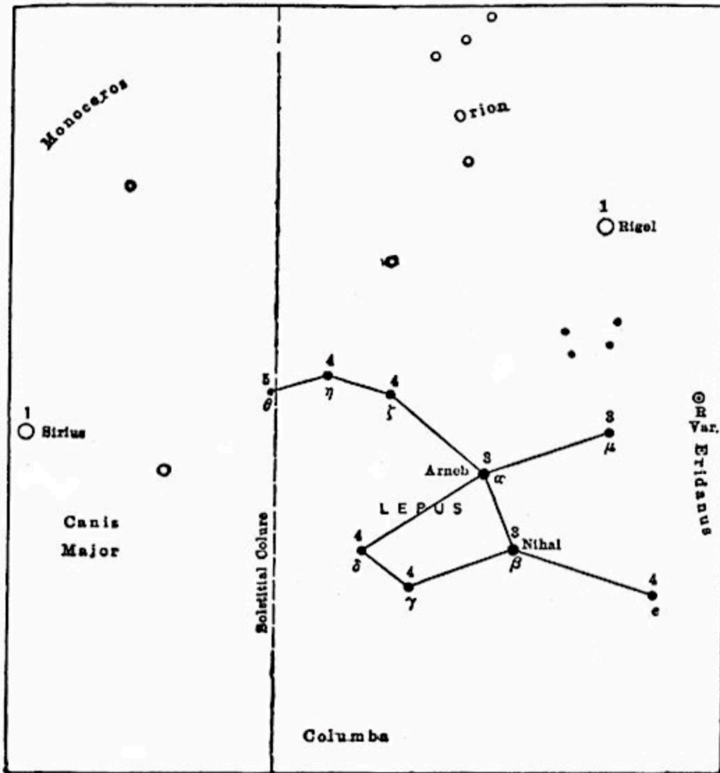
LEPUS
