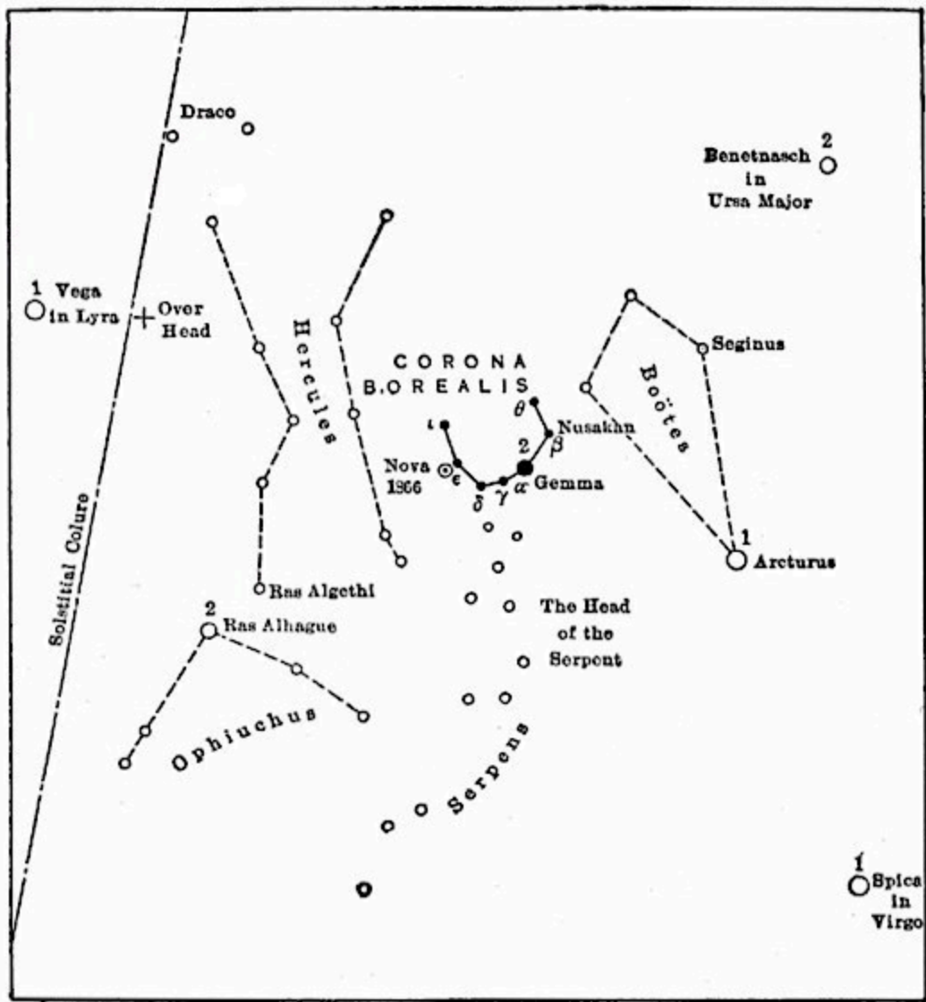
CORONA BOREALIS
