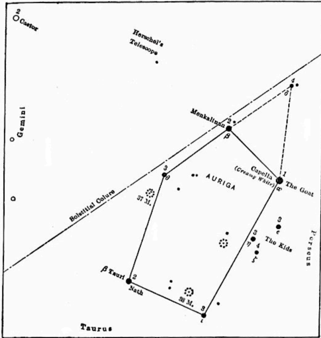
AURIGA
