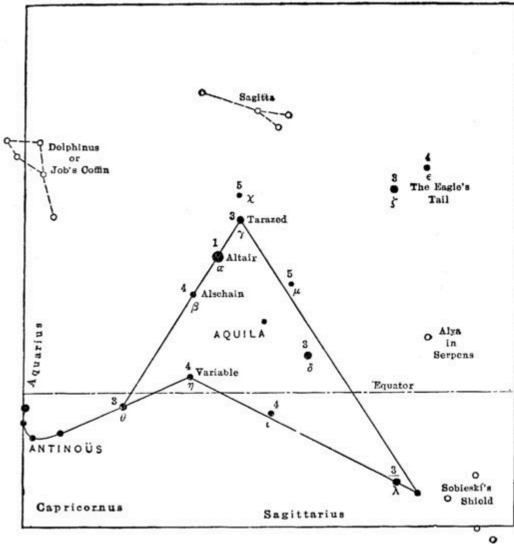
AQUILA & ANTINOÛS
