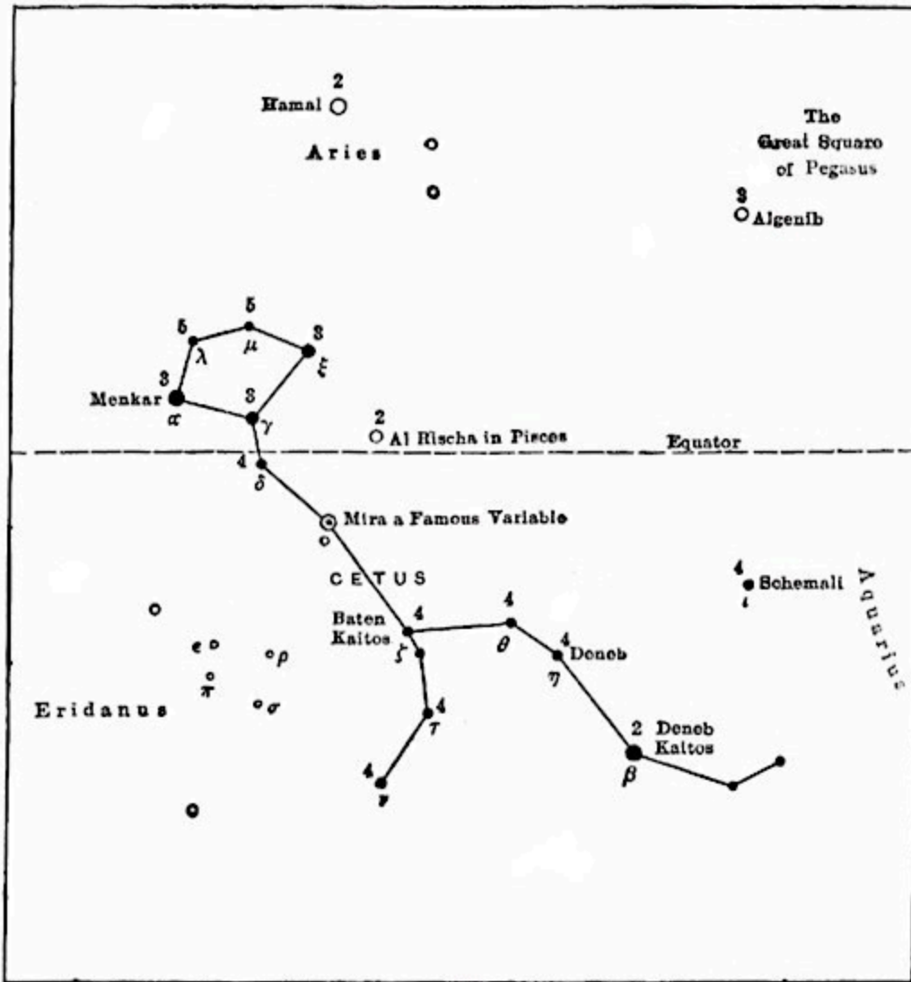
CETUS
