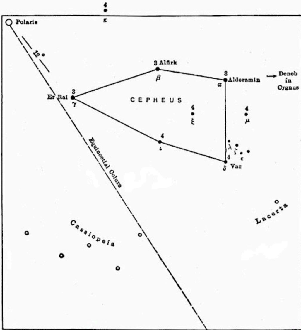
CEPHEUS
