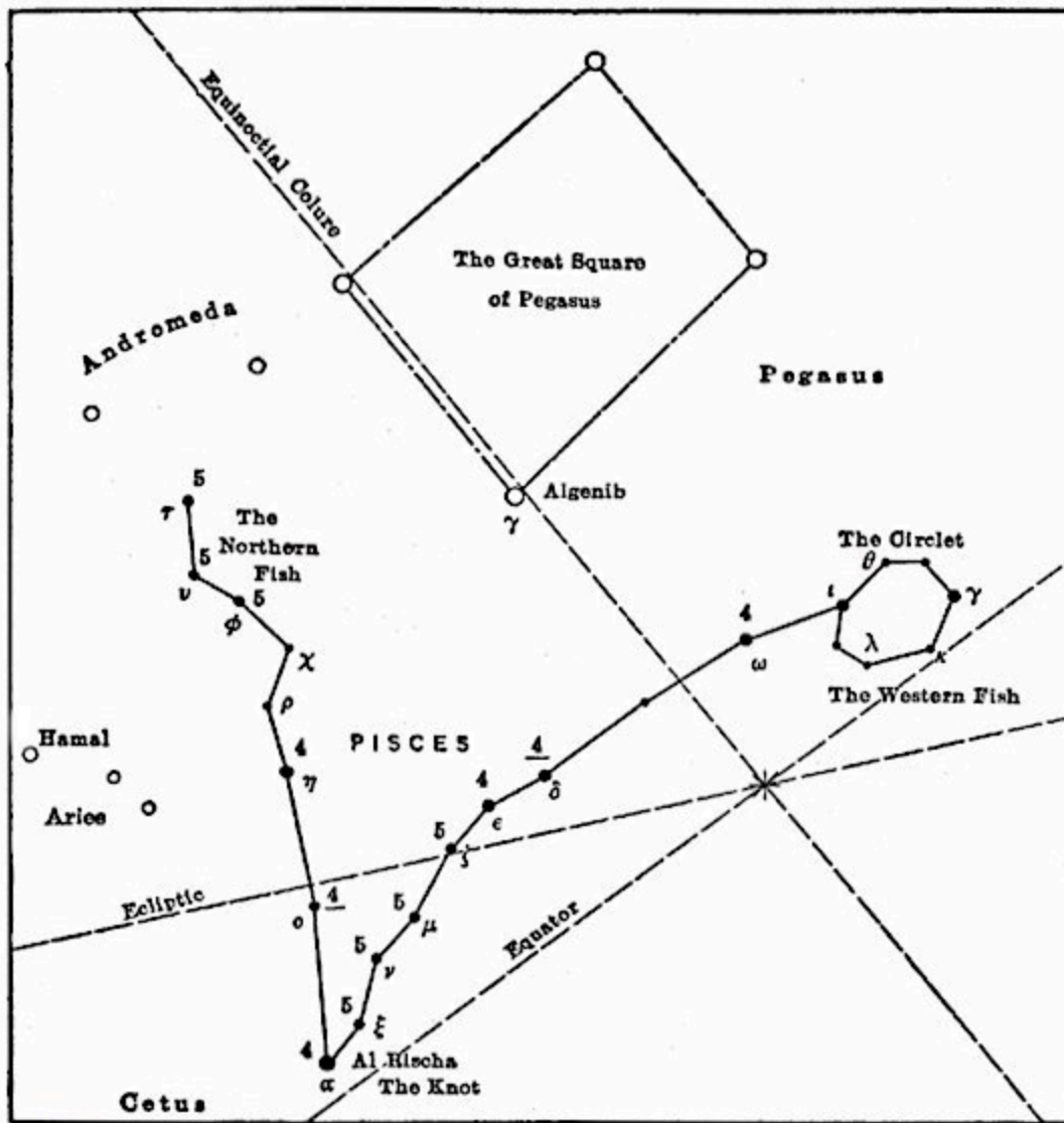
PISCES
