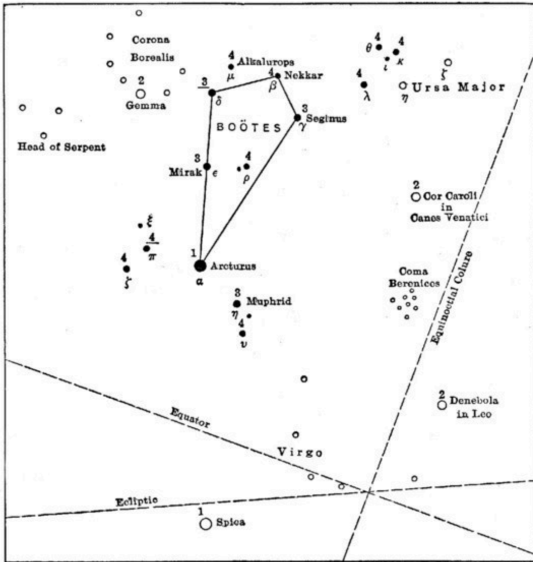
BOÖTES
