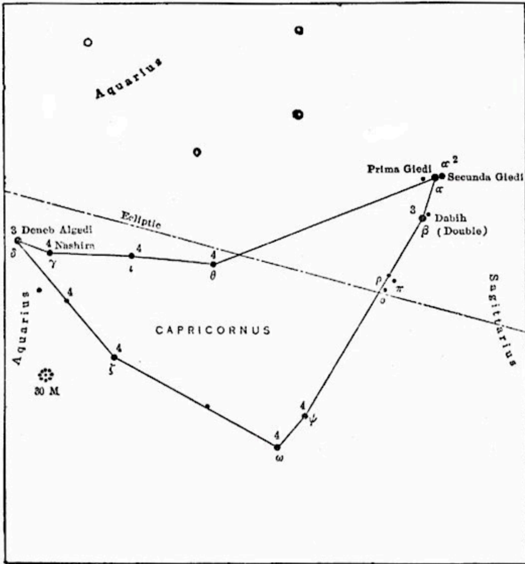
CAPRICORNUS
