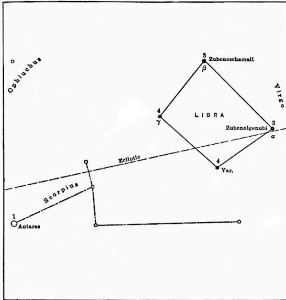
LIBRA
