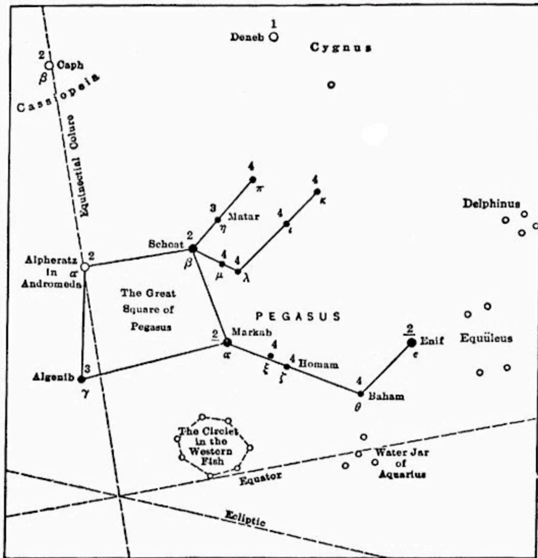
PEGASUS
