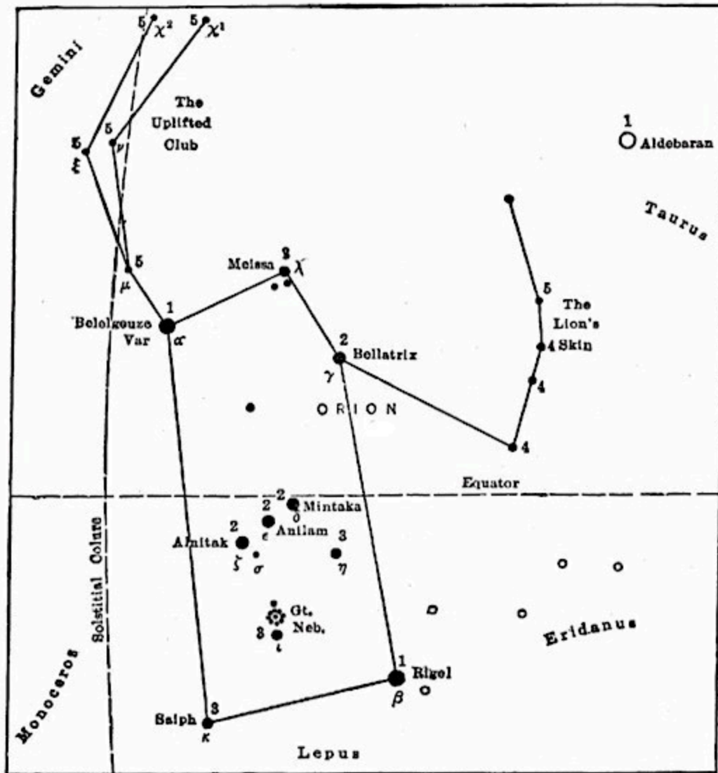
ORION
