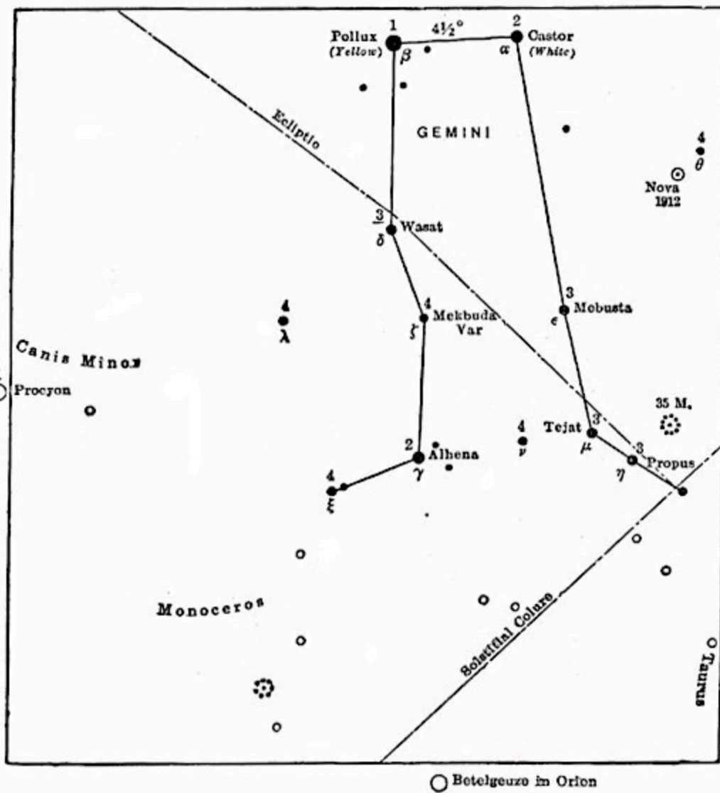
GEMINI
