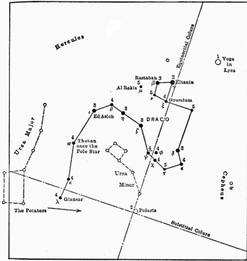
DRACO
