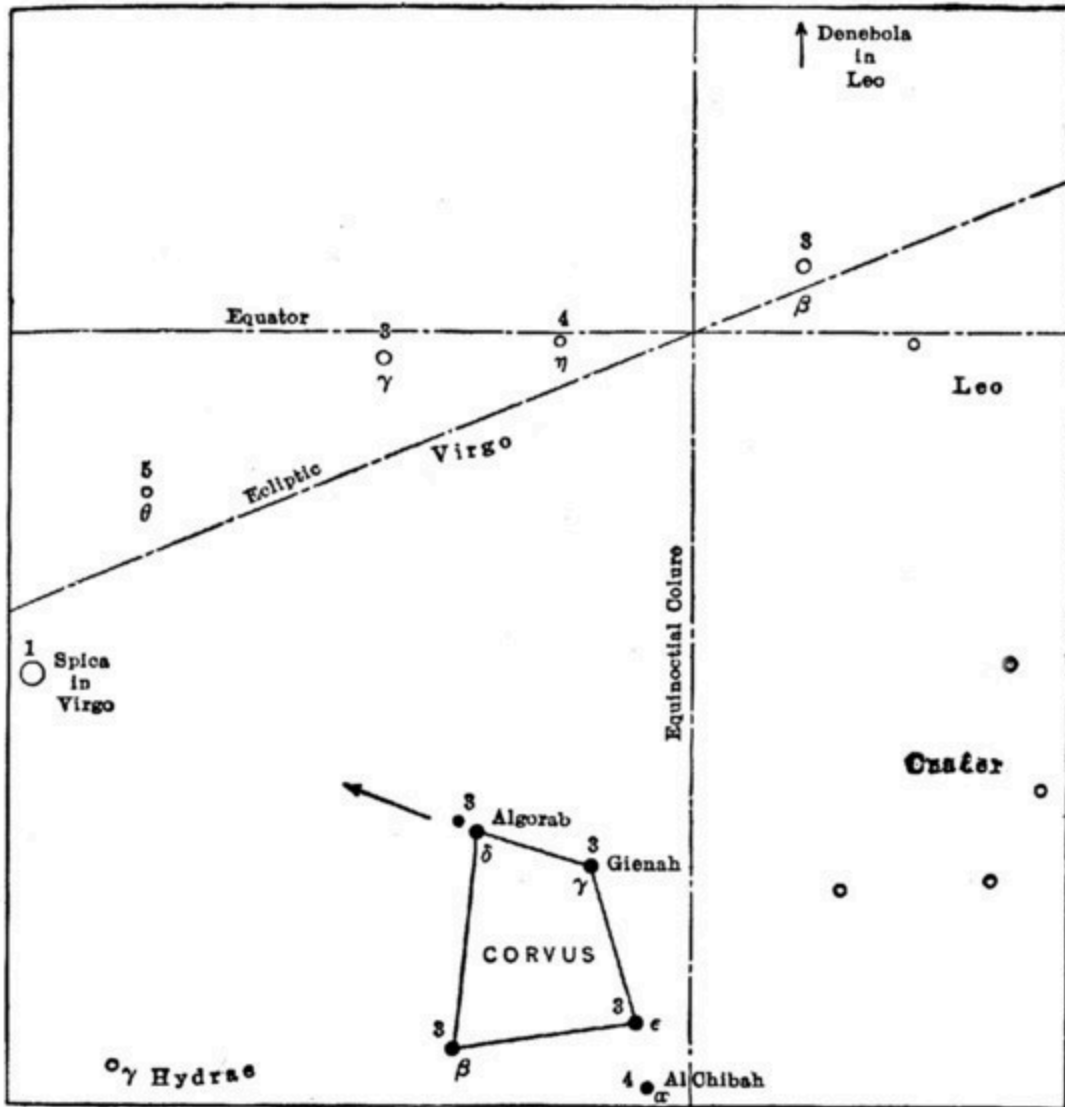
CORVUS
