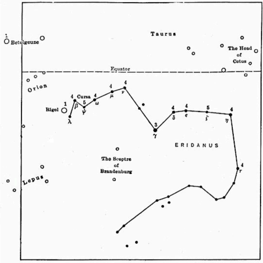
ERIDANUS
