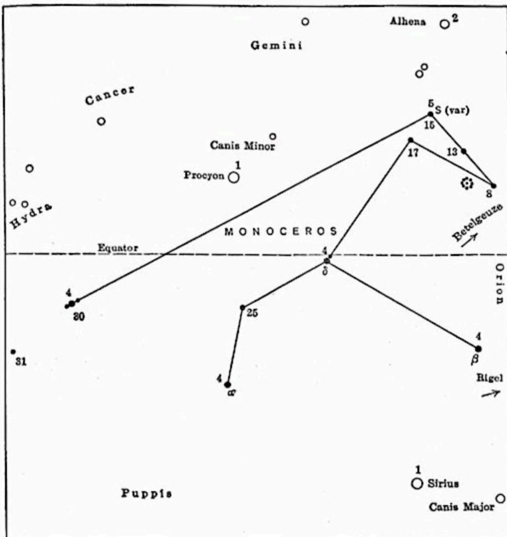
MONOCEROS
