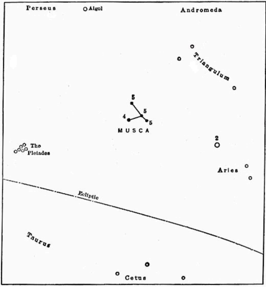
MUSCA
