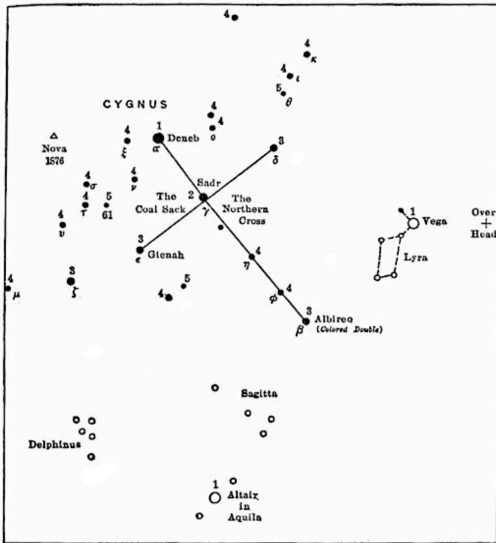
CYGNUS
