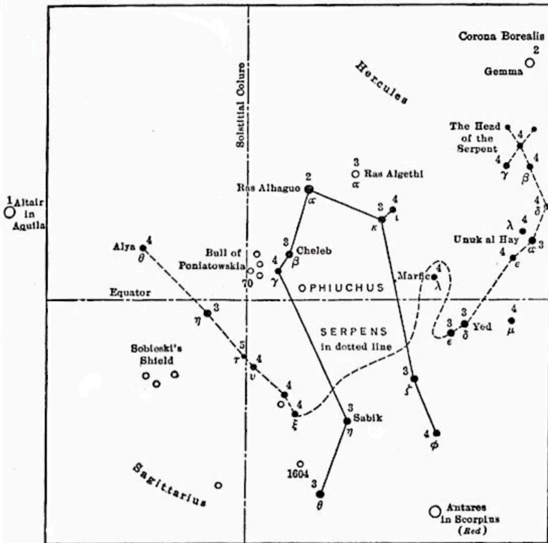
OPIUCHUS & SERPENS
